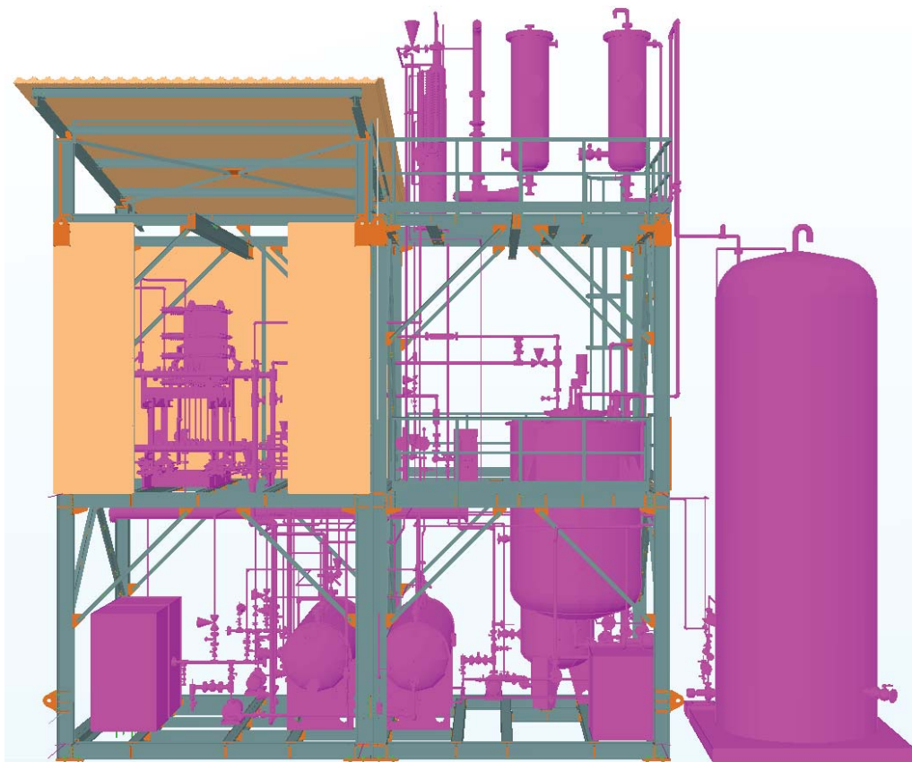
Figura 3 – Rappresentazione dell'impianto
