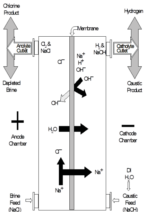
Figura 2 - Schema della cella elettrolitica
