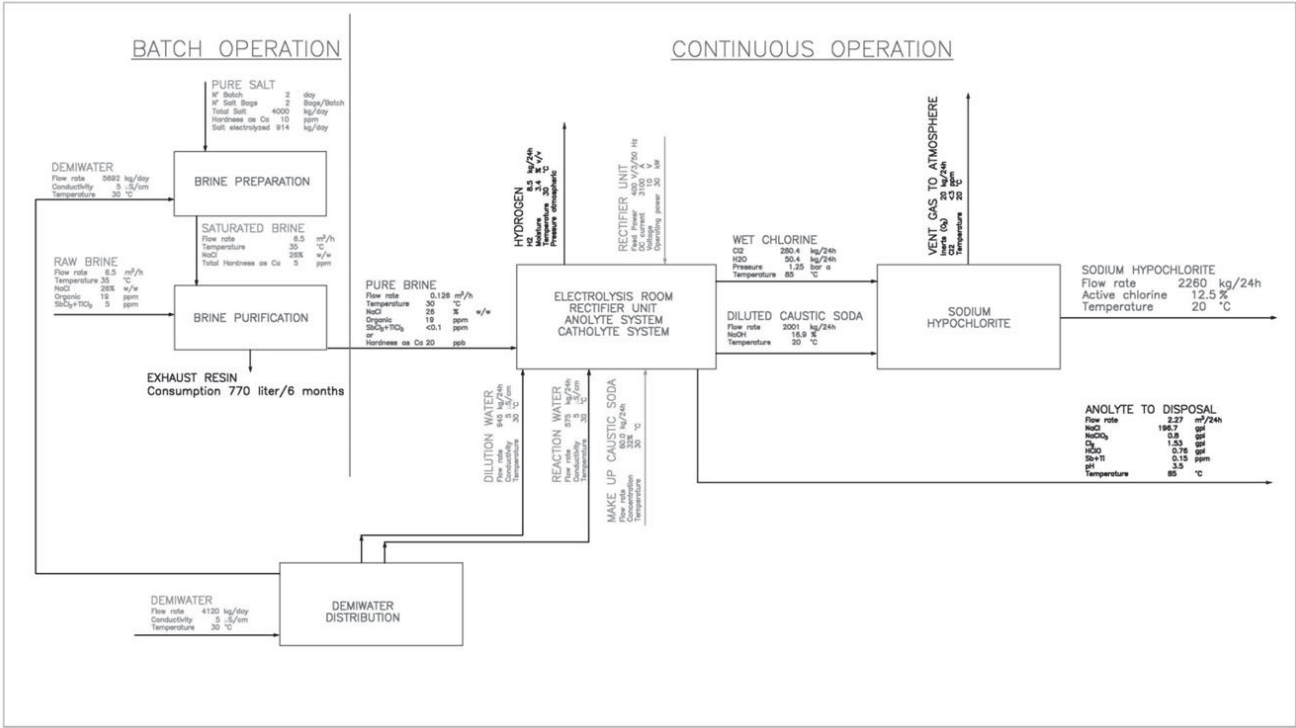
Figura 1 - Schema a blocchi del ciclo di recupero
